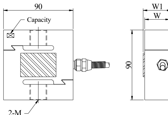
主視 (Front View)
